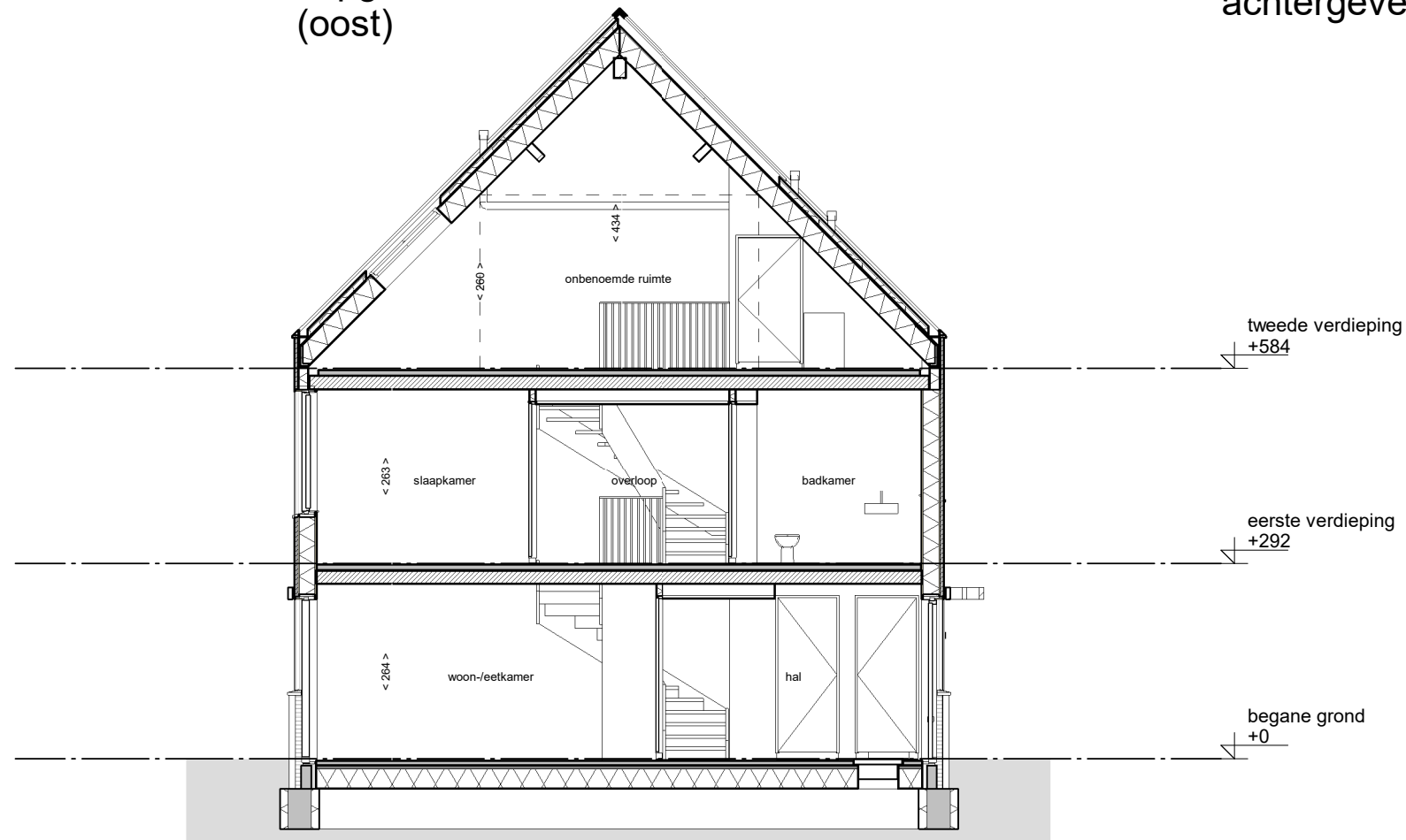
doorsnede
