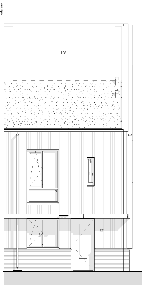
voorgevel (zuid)
